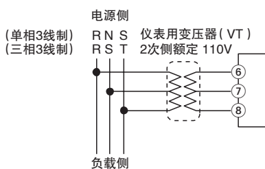
单相3线制/三相3线制
