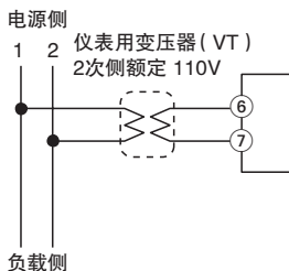
单相2线制
