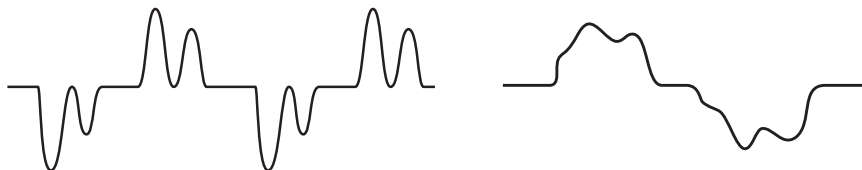
变频器一次侧电流波形示例
