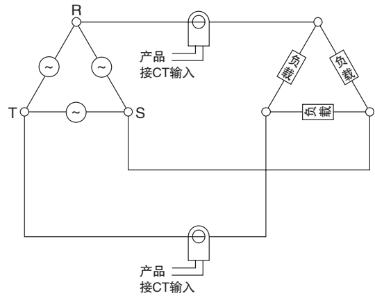
三相3线制(三角形接线)
