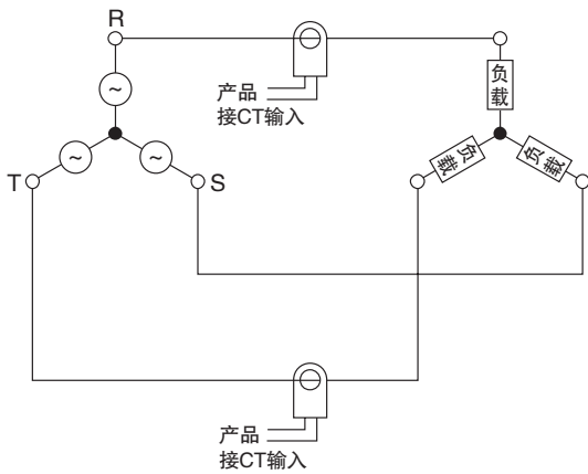
三相3线制(星形(Y)接线)
