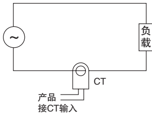
单相2线制
