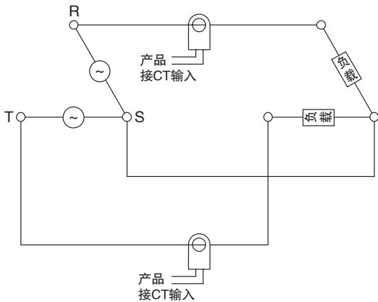
三相3线制(V形接线)
