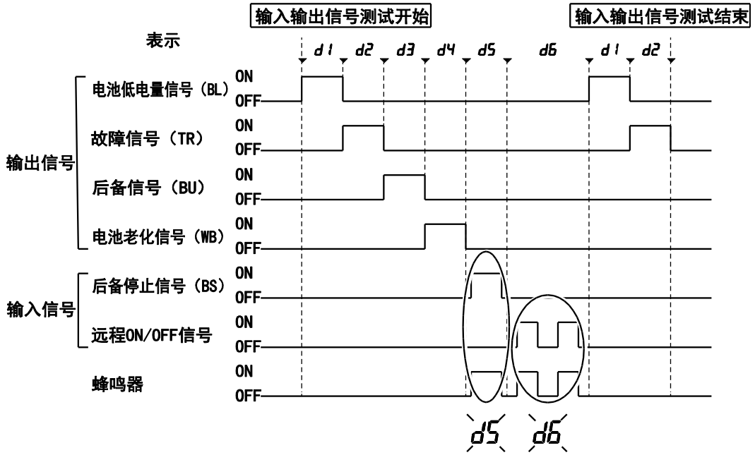
输入输出信号测试的操作图
