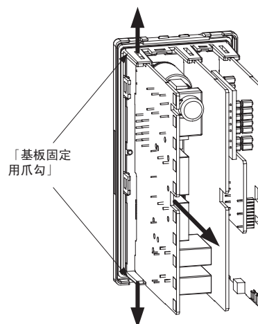
E5EN-H
