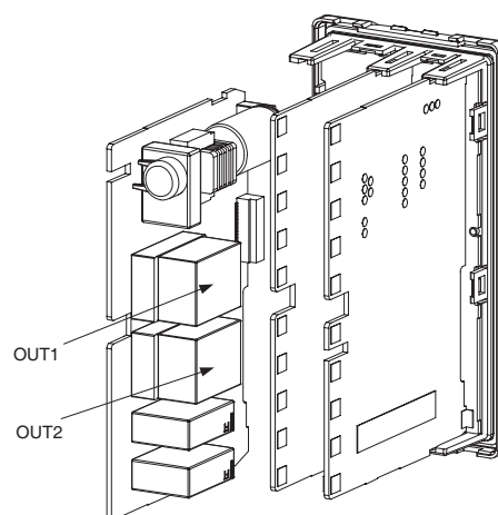
E5EN-H
