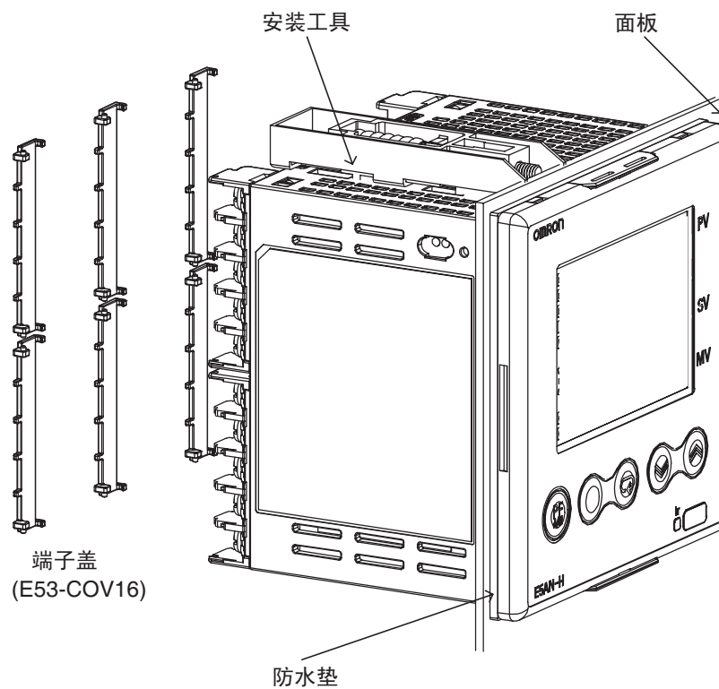
E5AN-H
