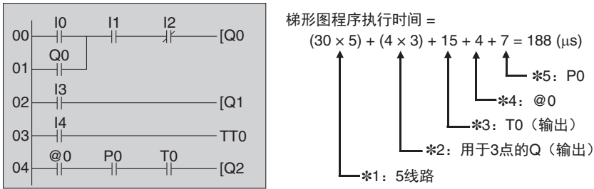
梯形图程序执行时间计算示例
