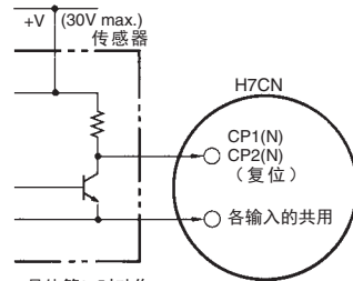
* 晶体管ON时动作
