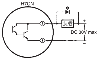
* 反电动势吸收用二极管
