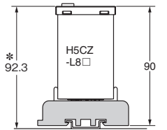
P2CF-08（-E）（另售）表面连接插座
