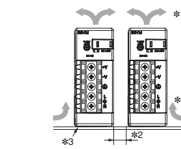
朝上安装
