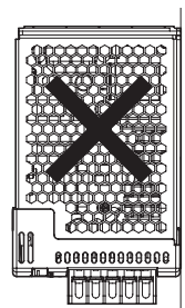
朝上安装方向的 侧面安装
