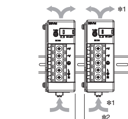
横向安装状态
