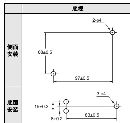
安装加工尺寸
