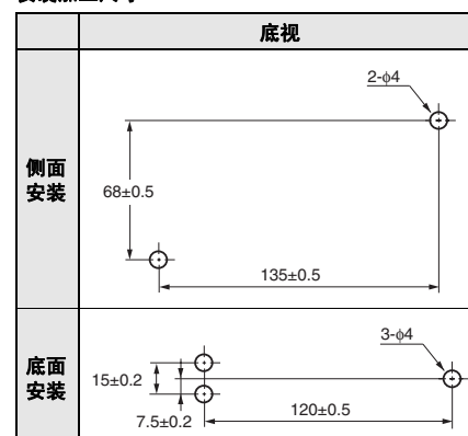
安装加工尺寸
