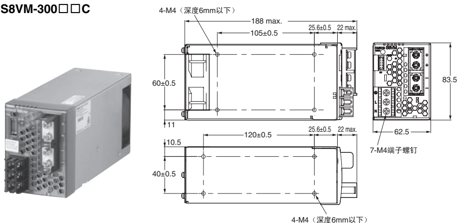
安装加工尺寸
