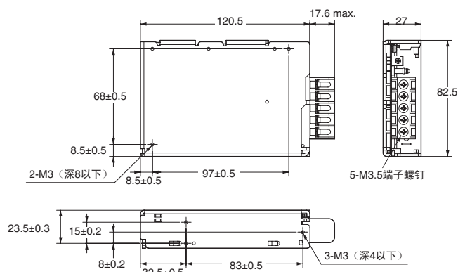
安装加工尺寸
