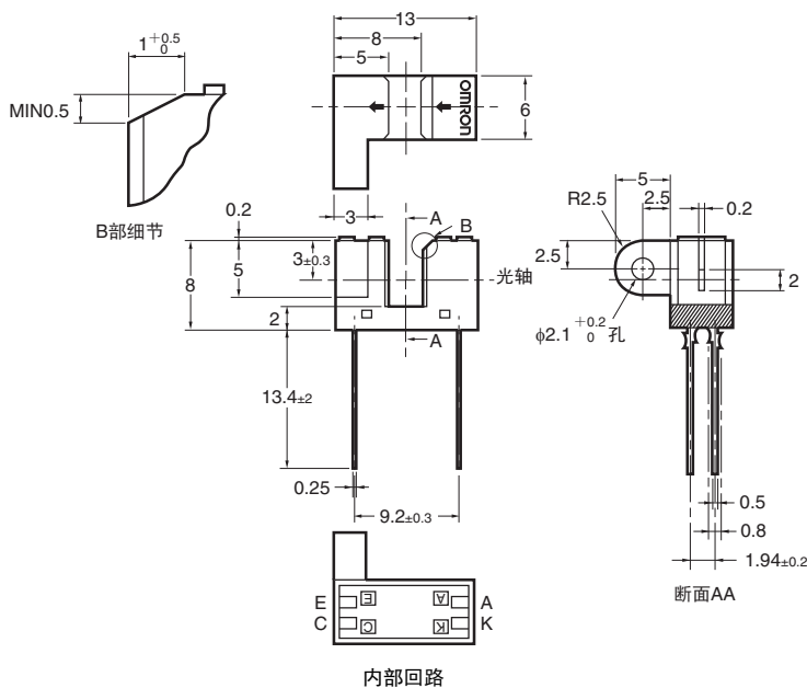
内部回路
