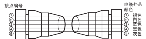
配线图 (5芯型)
