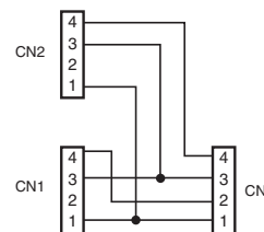
配线图
