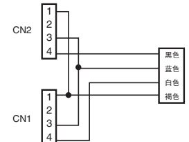
配线图
