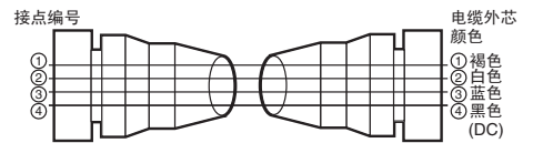
配线图 (4芯型)
