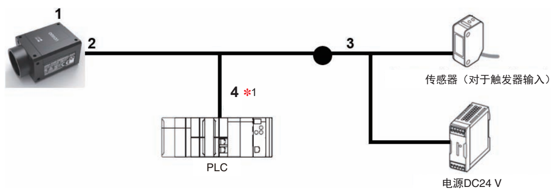
系统构成示例6：RS-232C结构
