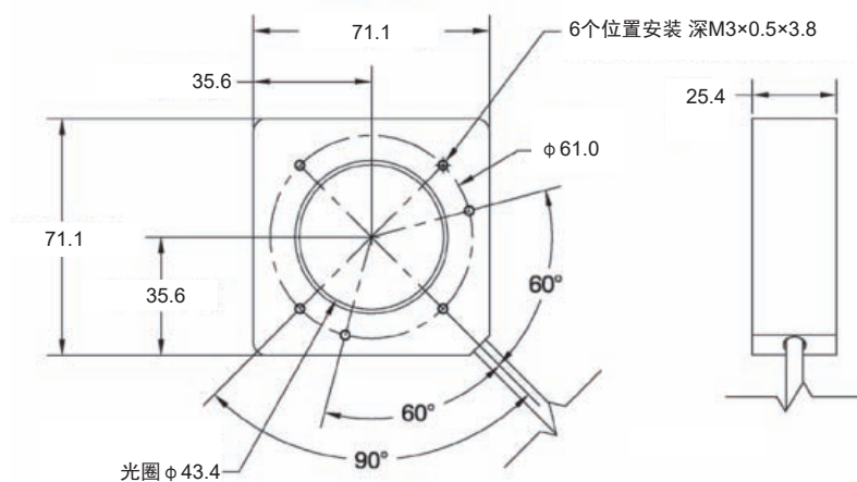
R-70环形照明
