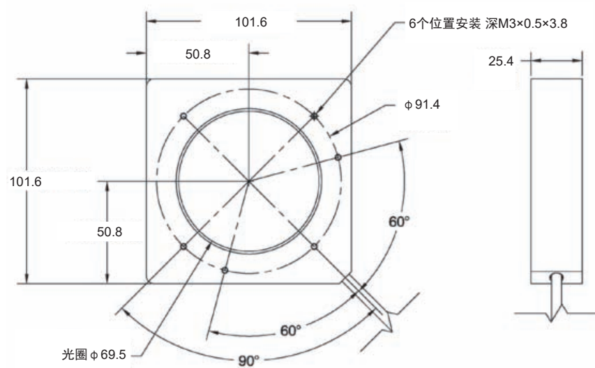
R-100环形照明
