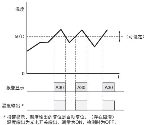
图 (3) (动作示意图)
