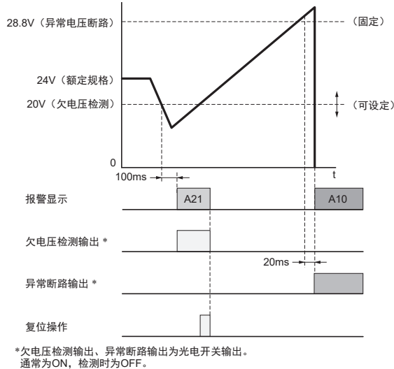
图 (1) (动作示意图)
