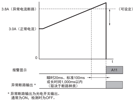
图 (2) (动作示意图)
