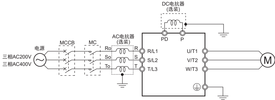
●连接示例
