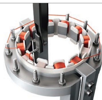
电机绕线工序
