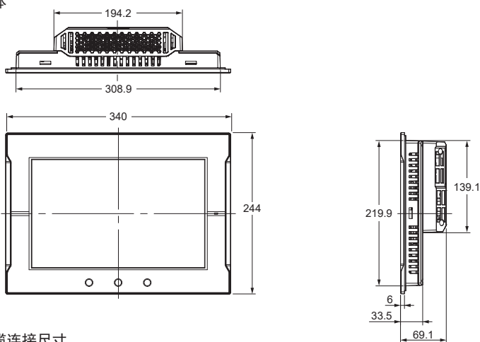
电缆连接尺寸
