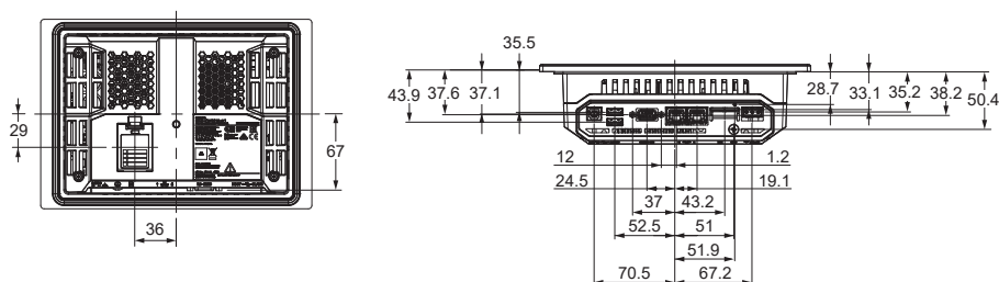
电缆连接尺寸
