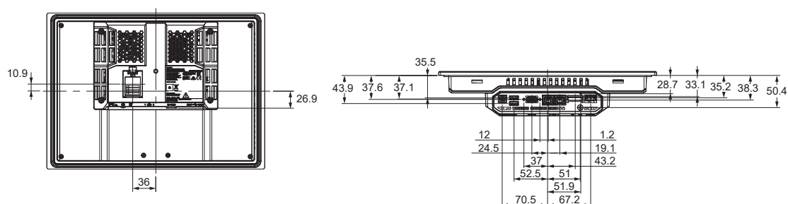
电缆连接尺寸
