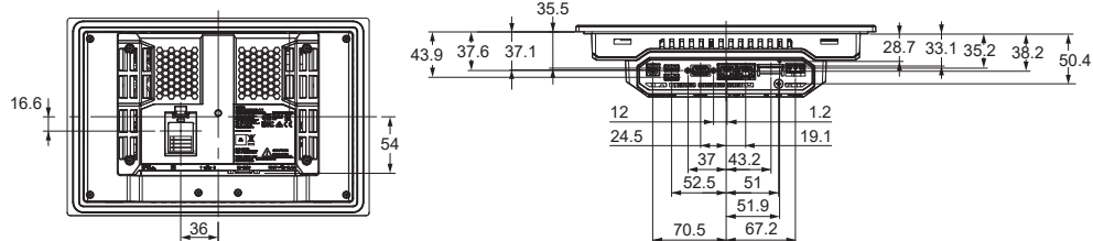
电缆连接尺寸
