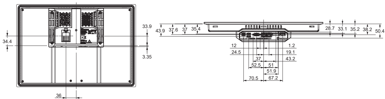
电缆连接尺寸
