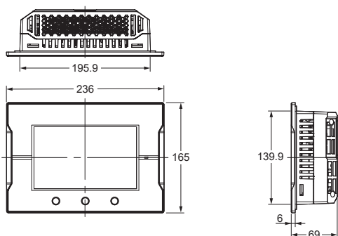
电缆连接尺寸
