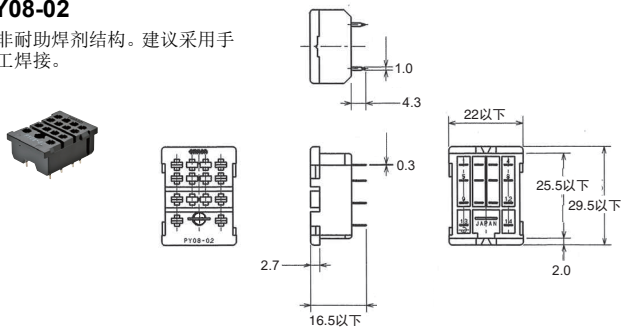
端子配置/内部连接图
