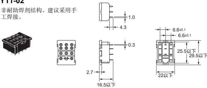
端子配置/内部连接图
