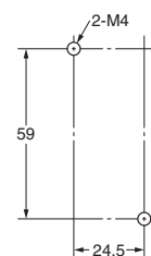
安装孔加工尺寸
