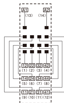
端子配置/内部连接图 (顶视图)
