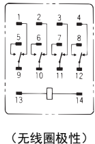
端子配置/内部连接图 (底视图) MY4(Z)H
