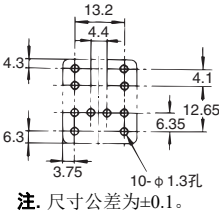
印刷电路板加工尺寸 (底视图)
