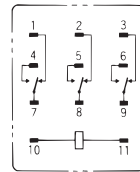
端子配置/内部连接图 (底视图) MY3
