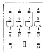
端子配置/内部连接图 (底视图) MY4
