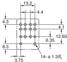
印刷电路板加工尺寸 (底视图)
