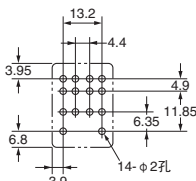
印刷电路板加工尺寸 (底视图)
