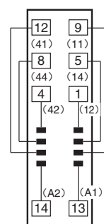
端子配置/内部连接图
