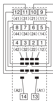
端子配置/内部连接图
