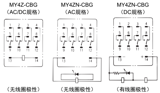
端子配置/内部连接图 (底视图)
