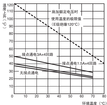
MY4 AC规格 50Hz
