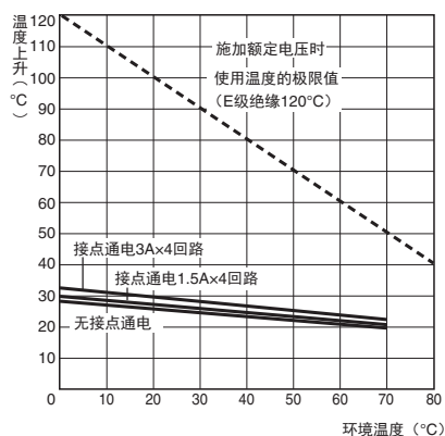
MY4 DC规格
