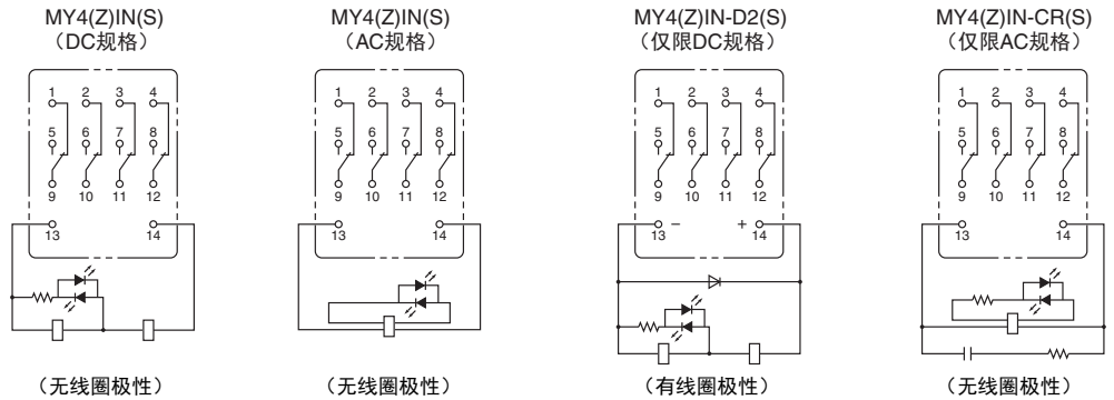
端子配置/内部连接图 (底视图)
