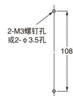
安装孔加工尺寸
