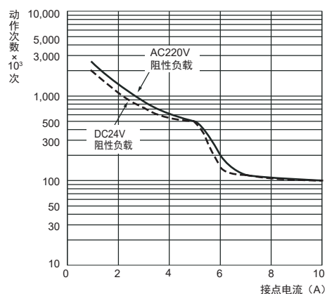
MY4□□-□□-GS-R (阻性负载)
