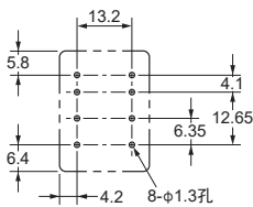
印刷电路板加工尺寸
