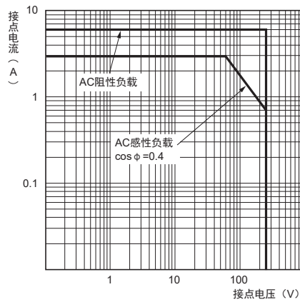
MY4□□-□□-GS-R（交流负载）
