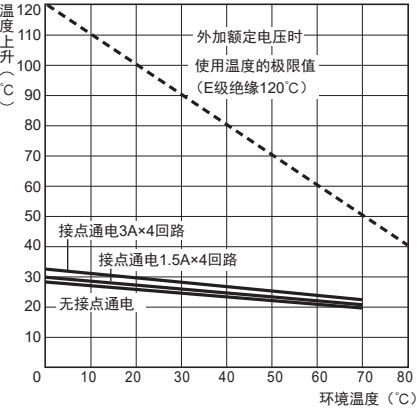
MY4□□-□□GS-R DC规格
