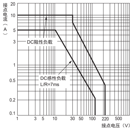
MY4□□-□□-GS-R（直流负载）
