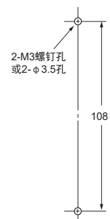
安装孔加工尺寸
