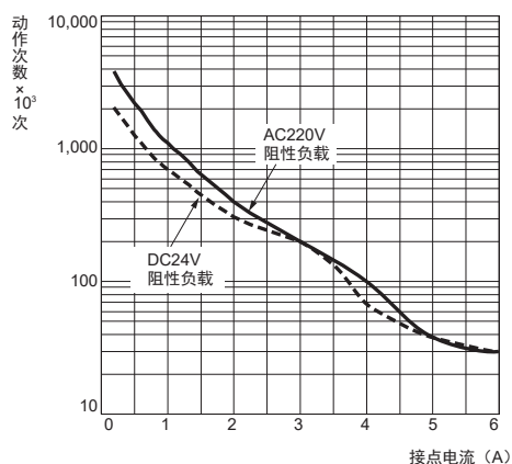
MY4□□-□□-GS-R (阻性负载)
