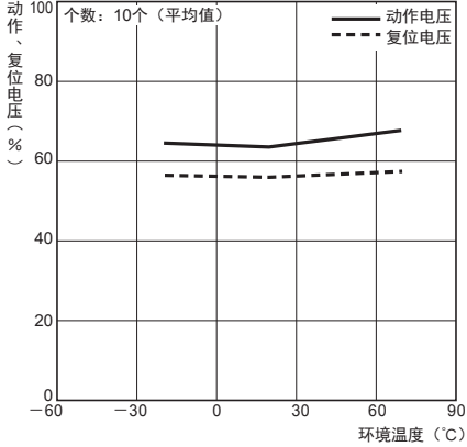
MY4□□-□□GS-R AC规格
