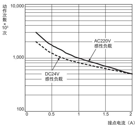
MY4□□-□□-GS-R (感性负载)
