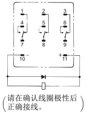
LY3-D
