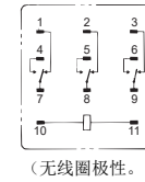
LY3
