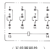
LY4
