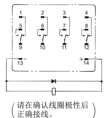
LY4-D
