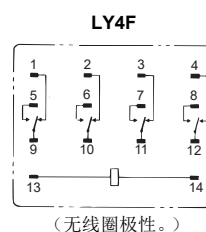
端子配置/内部连接图 (底视图)
