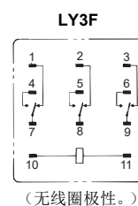
端子配置/内部连接图 (底视图)
