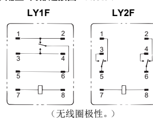
端子配置/内部连接图 (底视图)
