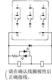
LY3N-D2
