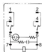
LY2 (Z) N-CR
