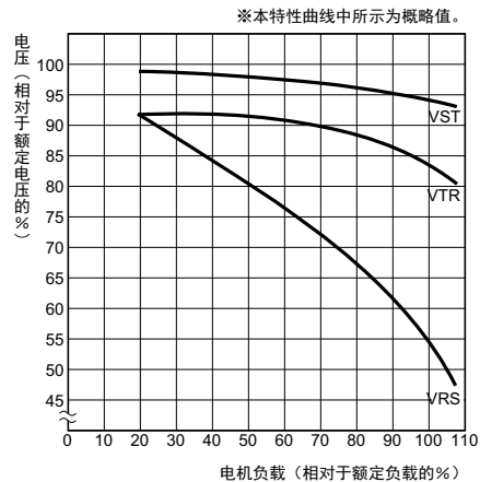
特性曲线（图）
