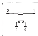
端子配置/内部连接图 (TOP VIEW)
