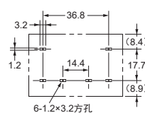
印刷基板加工尺寸 (BOTTOM VIEW) 尺寸公差为±0.1mm。
