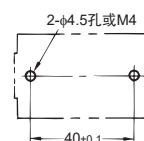
安装孔加工尺寸
