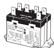
G7L-2A-TUBJ (带测试按钮)
