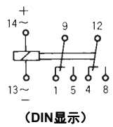
(DIN显示)
