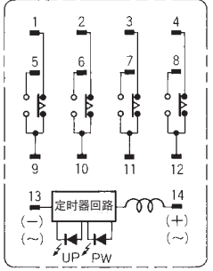
(底视图)
