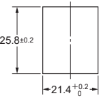
安装孔加工尺寸
