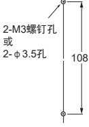
安装孔加工尺寸
