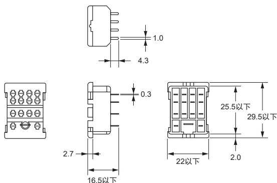
端子配置/内部连接图
