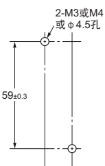
(顶视图)
