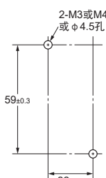
(顶视图)
