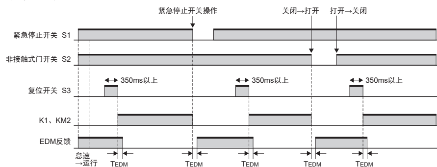
动作时序图
