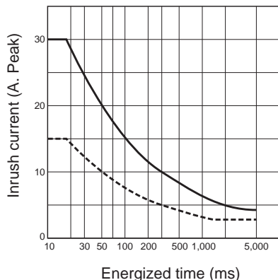
G3TA-OA202SZ/OA202SL-US
