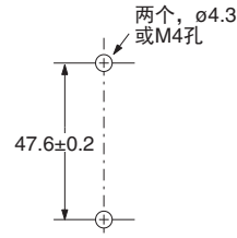
安装孔
