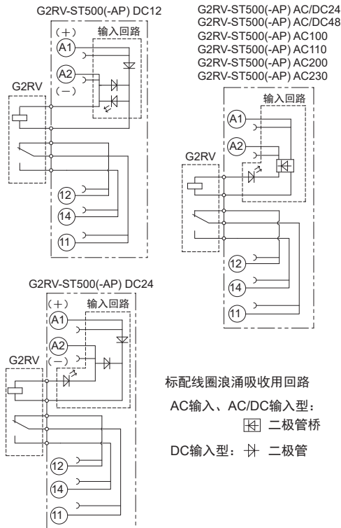
端子配置/内部连接图 (顶视图)
