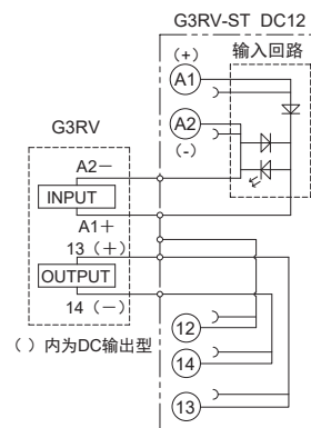
端子配置/内部连接图 (顶视图)
