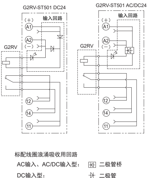
端子配置/内部连接图 (顶视图)
