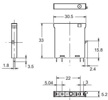
G3RV-202S(L)
