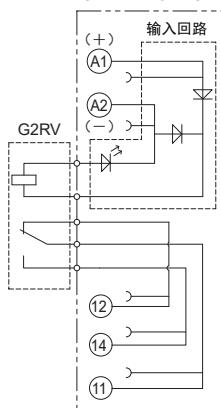
端子配置/内部连接图 (顶视图)
