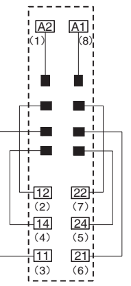
端子配置/内部连接图 (顶视图)
