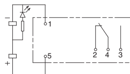
端子配置/内部连接图 (底视图)
