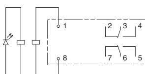
端子配置/内部连接图 (底视图)
