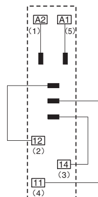
端子配置/内部连接图 (顶视图)
