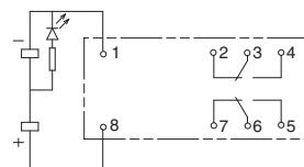
端子配置/内部连接图 (底视图)
