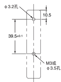
安装孔加工尺寸
