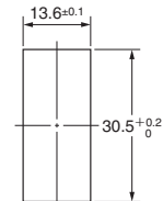
安装孔加工尺寸 (底视图)
