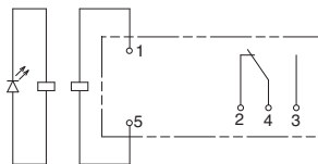
端子配置/内部连接图 (底视图)
