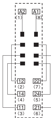
端子配置/内部连接图 (顶视图)
