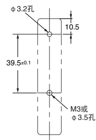
安装孔加工尺寸
