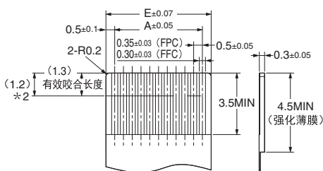
推荐FPC / FFC尺寸
