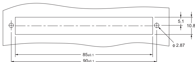
面板加工尺寸 (顶视图)
