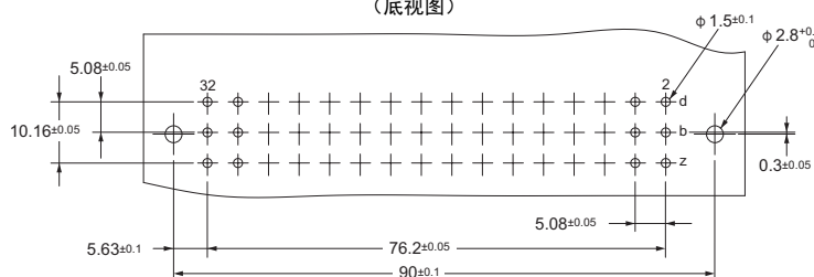
印刷电路板加工尺寸 （底视图）
