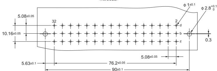
印刷电路板加工尺寸 （底视图）
