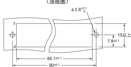
面板加工尺寸 （顶视图）
