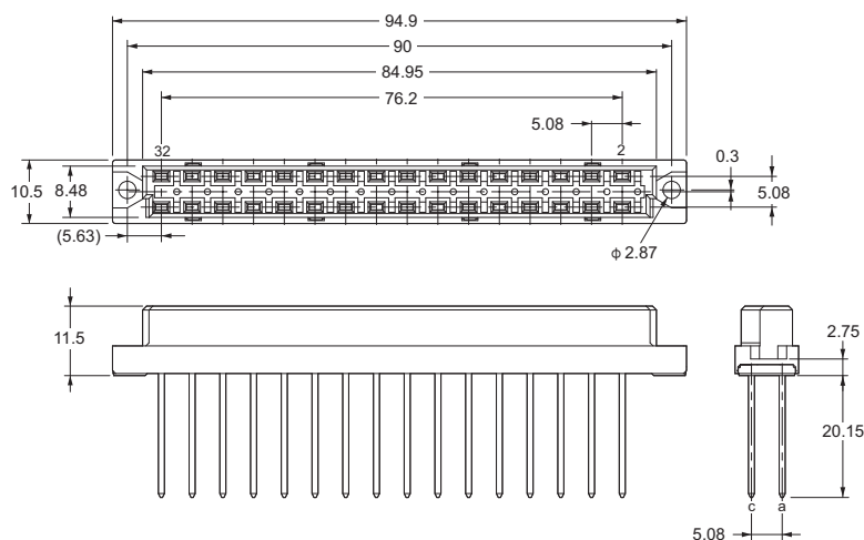
印刷电路板加工尺寸 (底视图)
