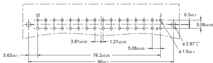
面板加工尺寸 (顶视图)
