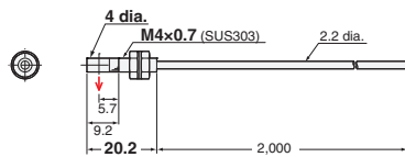
33-H E32-T81R-S 2M (No Cutting) + E39-F2
