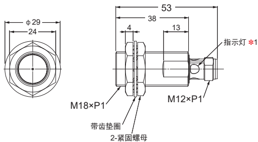
E2E-X7D□-M1/-M1G
