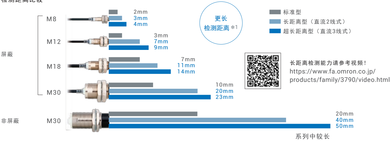
检测距离比较
