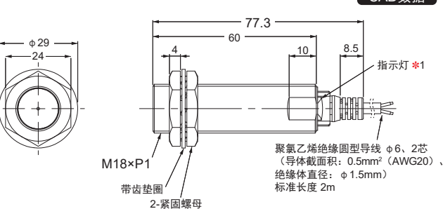
E2E-X10D□L
