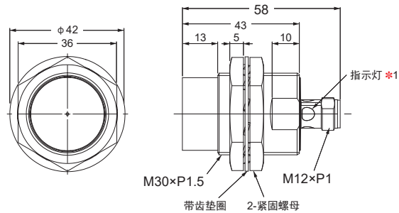
E2E-X20MD□-M1/-M1G
