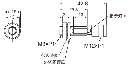
E2E-X3D□-M1/-M1G
