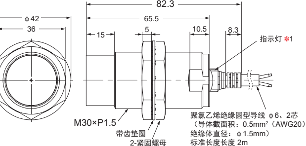
E2E-X30MD□L
