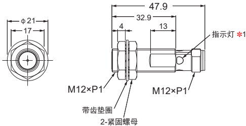
E2E-X7D□-M1/-M1G
