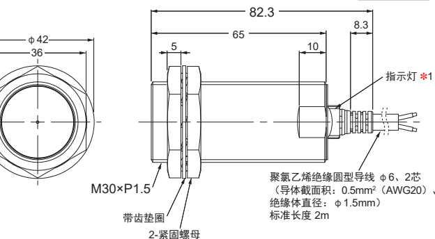
E2E-X10D□L
