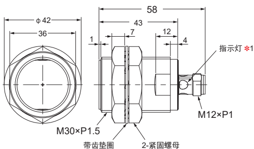
E2E-X□30-M1
