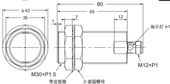
E2E-X□L30-M1
