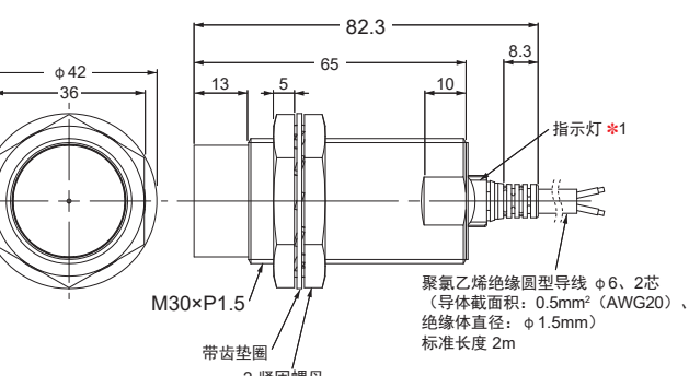
E2E-X30MD□L
