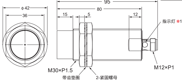
E2E-X50M□L30-M1
