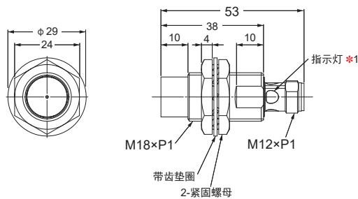
E2E-X14MD□-M1/-M1G
