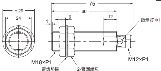
E2E-X□L30-M1
