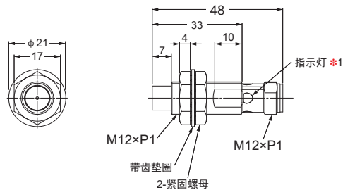
E2E-X14MD□-M1/-M1G
