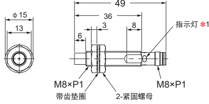
E2E-X□M□L8-M1
