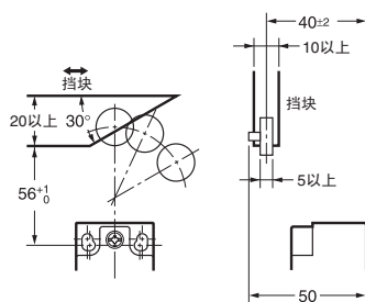
密封柱塞型 (D4N-□□31R)
