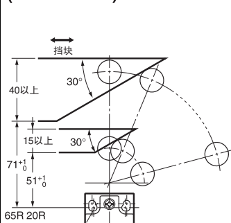
可调滚珠摆杆，锁定型 (金属摆杆，树脂滚珠) (D4N-□□2GR)
