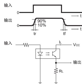
图9. 应答时间测定回路
