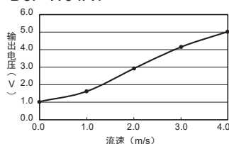
D6F-W04A1
