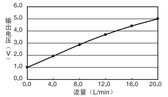
D6F-20A6-000 D6F-20A61-000
