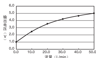
D6F-10A5-000
