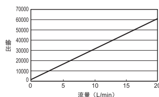
D6F-20A7D-000-0
