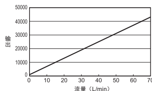
D6F-70AB71D-000-0
