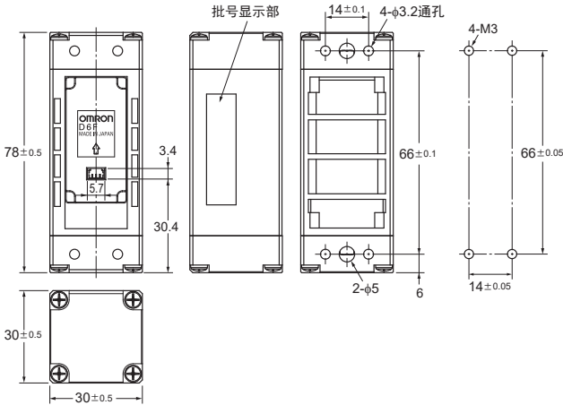
安装孔加工尺寸
