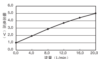
D6F-20A5-000
