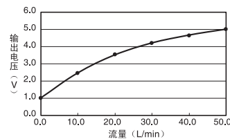
D6F-50A6-000 D6F-50A61-000
