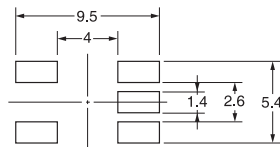
印刷基板焊盘尺寸 (TOP VIEW)
