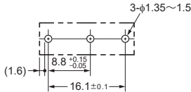
<印刷基板用端子孔加工图(参考)>
