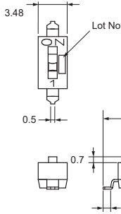
1极开关外形尺寸
