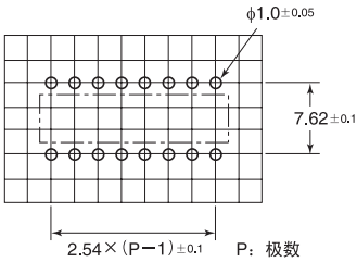
印刷基板加工尺寸 (TOP VIEW)
