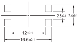
印刷基板焊盘尺寸示例 (TOP VIEW) (基板 t=1.6)
