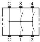
内部接线图(TOP VIEW)
