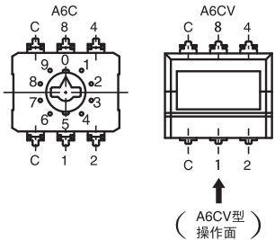
端子配置
