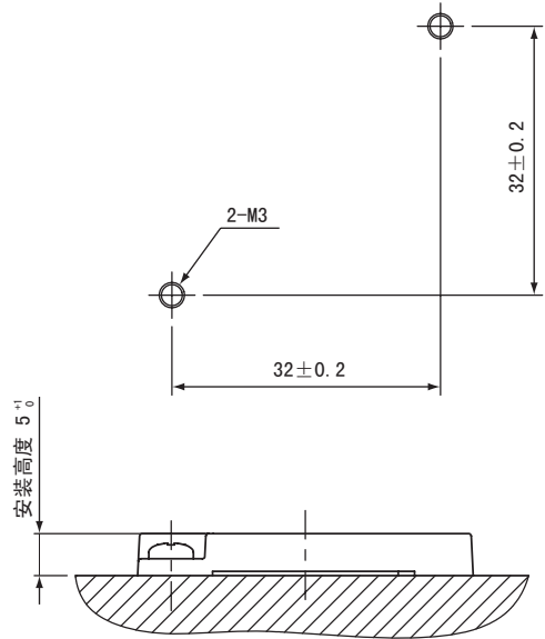
安装孔加工尺寸
