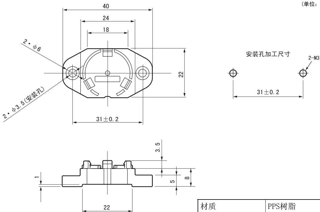
V700-A80 (附件)
