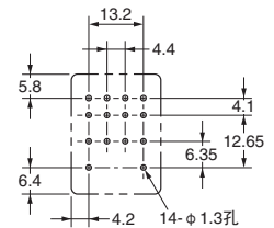
印刷电路板加工尺寸
