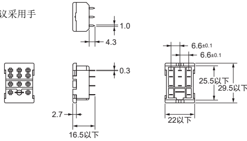
端子配置/内部连接图
