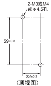
安装孔加工尺寸
