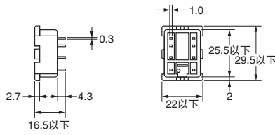
端子配置/内部连接图
