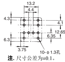
印刷电路板加工尺寸 (底视图)
