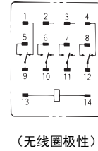
端子配置/内部连接图 (底视图) MY4(Z)H
