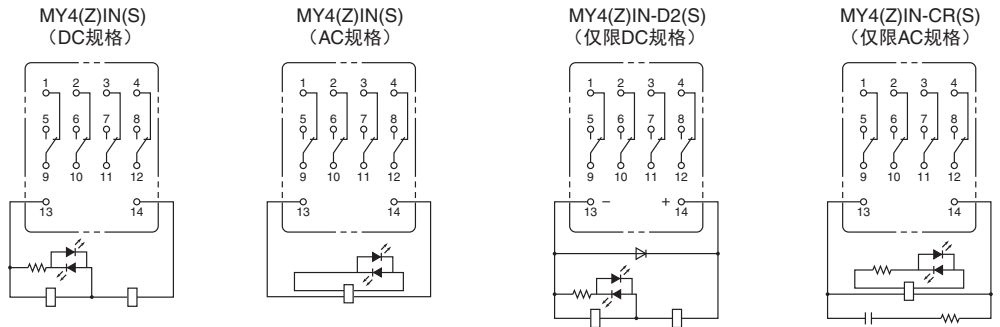
端子配置/内部连接图 (底视图)
