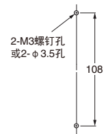
安装孔加工尺寸
