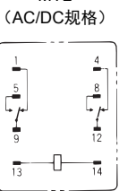
端子配置/内部连接图 (底视图) MY2
