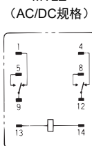
端子配置/内部连接图 (底视图) MY2Z
